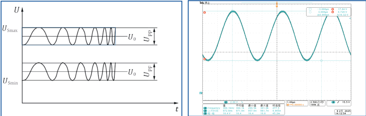
图4-发电机纹波叠加测试脉冲频率时序
