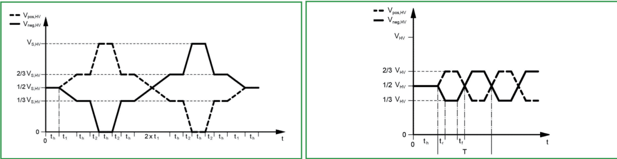
高压电压偏移测试的测试步骤1的高压电压曲线
