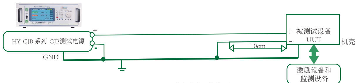
图HDC104-1 脉动试验系统典型配置
