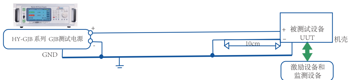
图LDC103-1 电压畸变频谱试验系统典型配置1
