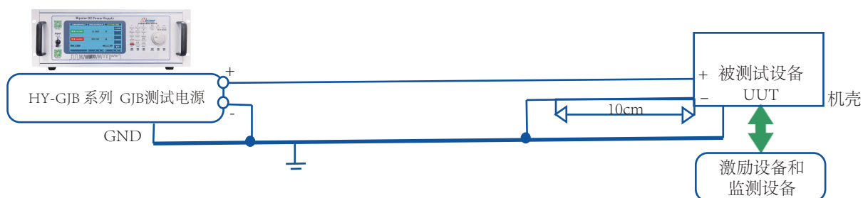
图LDC102-1 正常稳态电压试验系统典型配置
