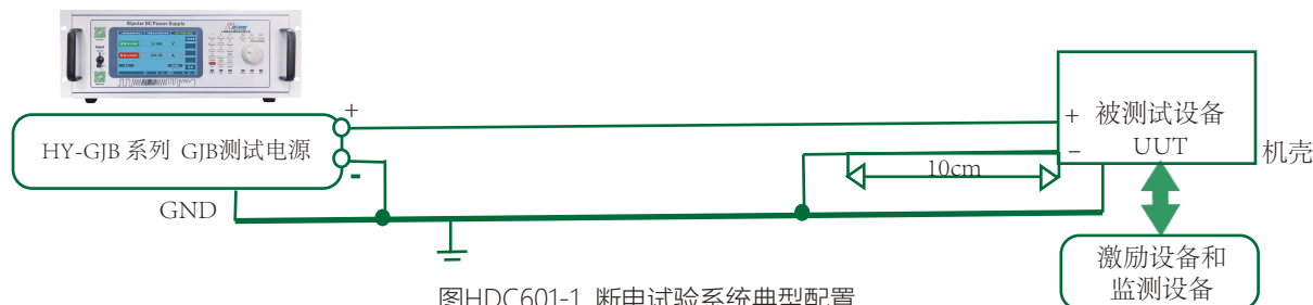
图HDC601-1 断电试验系统典型配置
