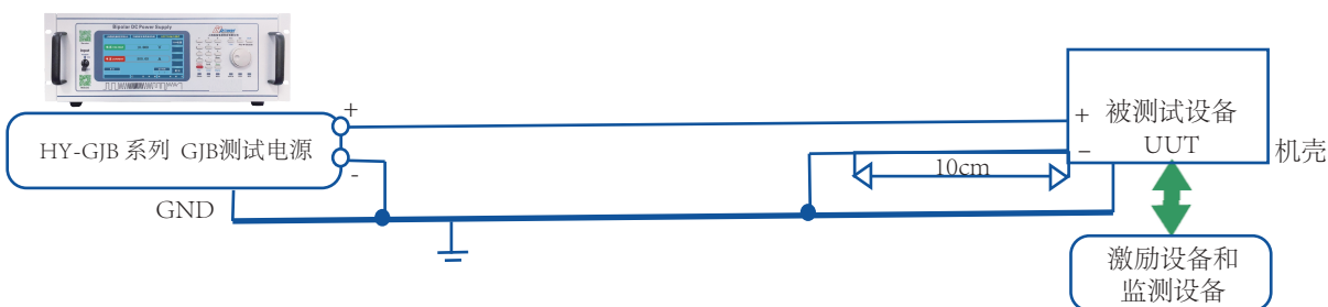
图LDC501-1 起动电压瞬变试验系统典型配置
