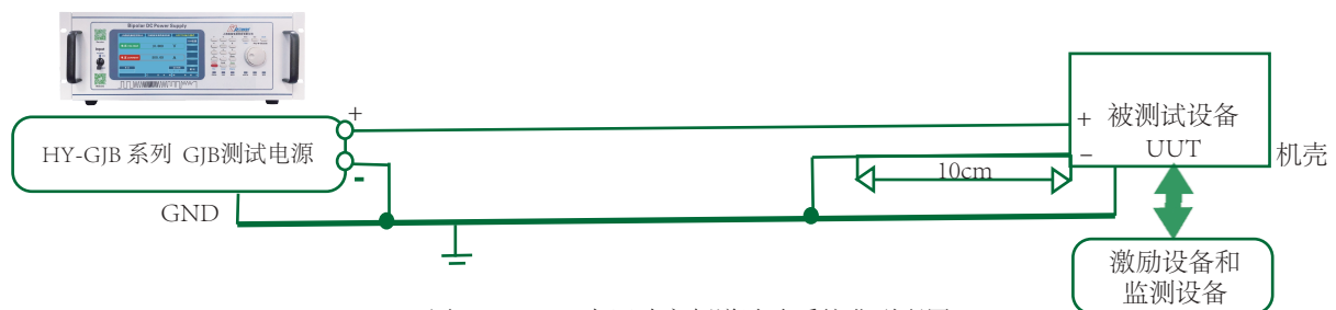
图HDC103-1 电压畸变频谱试验系统典型配置1
