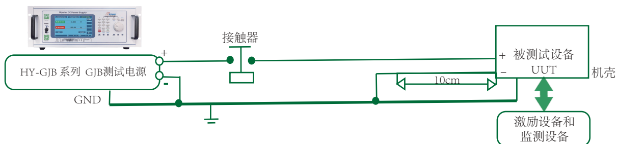
图HDC201-1 供电转换中断试验系统典型配置
