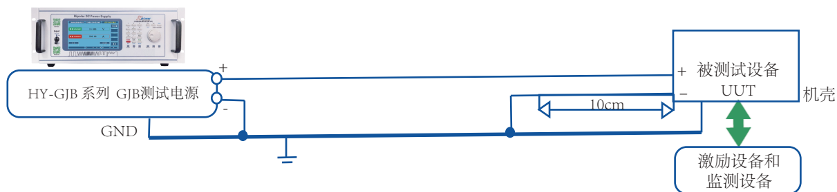
图LDC401-1 应急稳态电压试验系统典型配置
