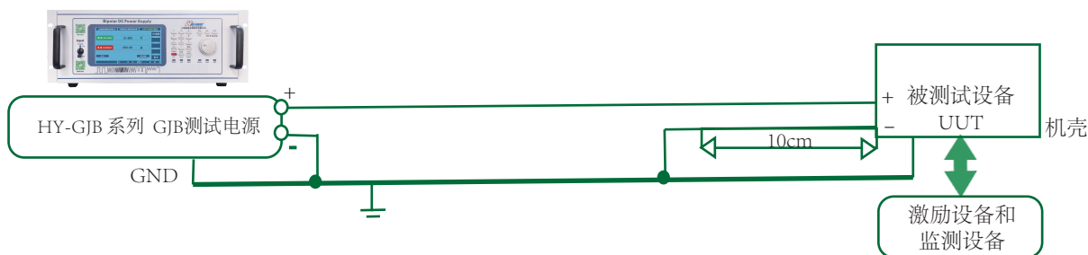
图HDC301-1 非正常稳态电压试验条件
