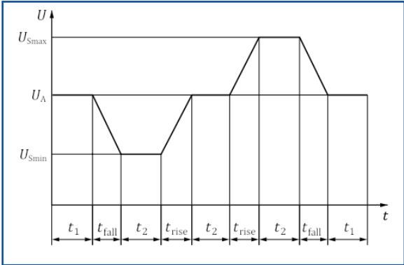
图1——直流电源电压测试曲线
