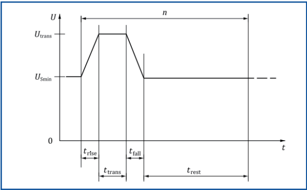
图2-在室温和Tmin下测试启动试验波形图
