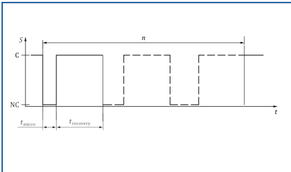
图10-12V/24V电力系统下可变中断的微中断 (UN)
