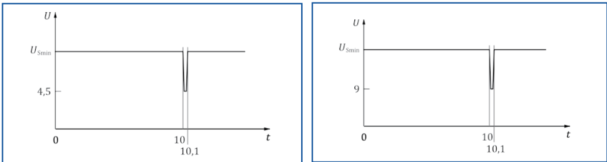
图7-12V电力系统短电压降 图8-24V电力系统短电压降
