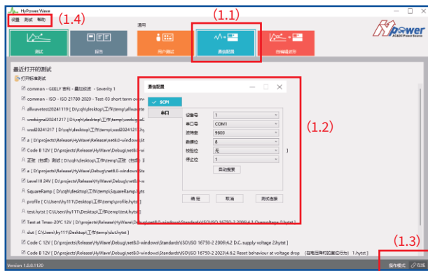
(图1:主界面和连接通讯)
